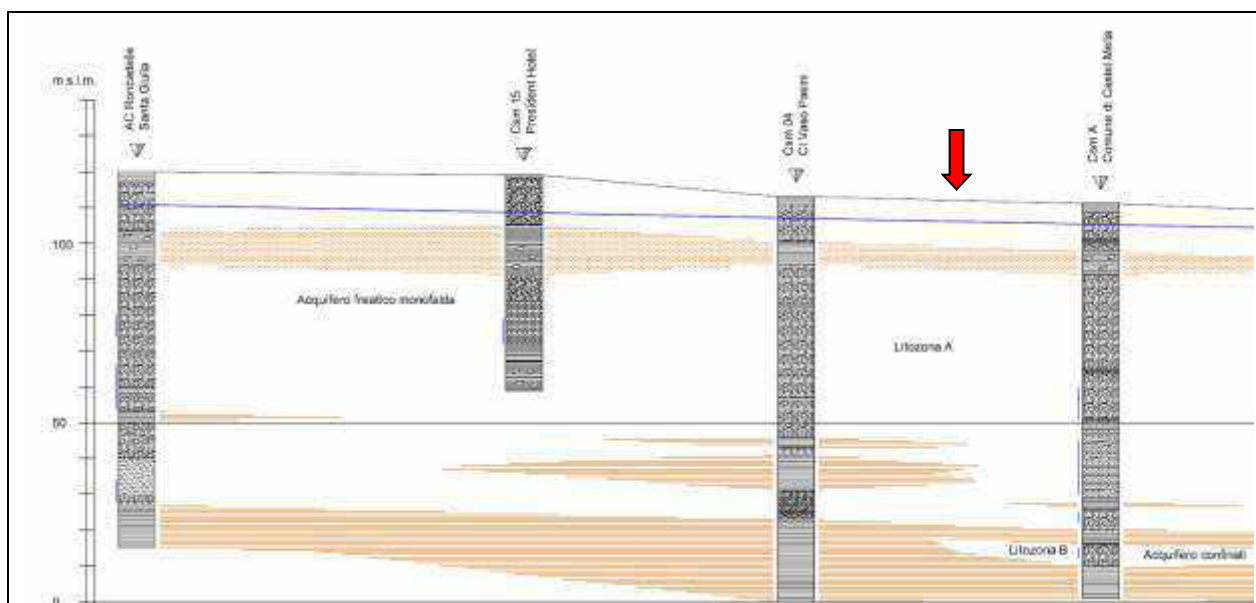
Figura 8 – Sezione stratigrafica AA' (da PGT)
