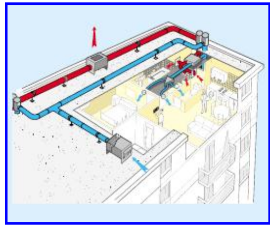
Impianto di ventilazione meccanica forzata con recuperatore di calore
