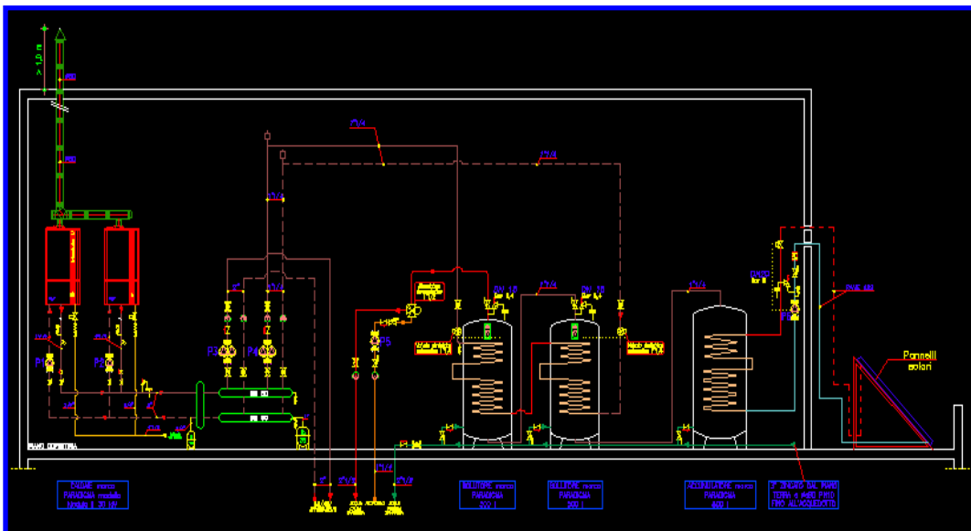
Progetto di sistema con caldaie a condensazione e integrazione pannelli solari
