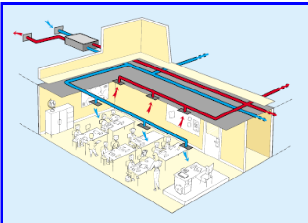
Impianto di ventilazione meccanica forzata con recuperatore di calore
